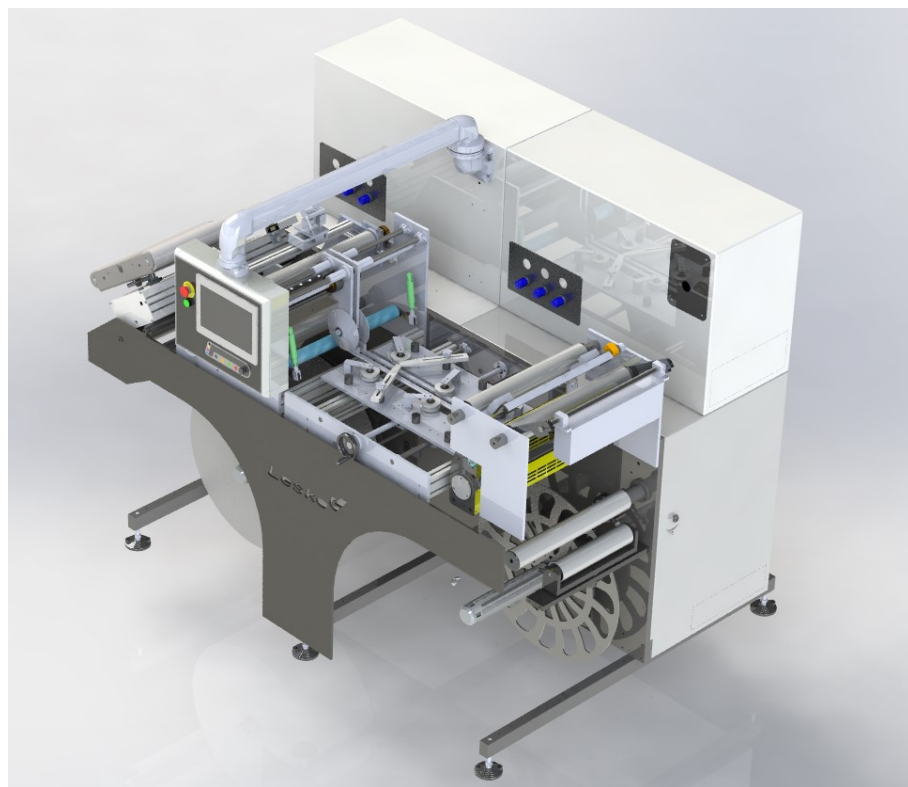
Neuentwicklung von Lesko: Maschine zum Verschließen von Shrink Sleeves
